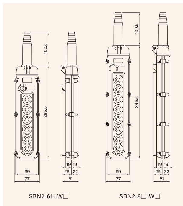
型式 SBN2-6H-WA 制御停止釦付ペンダントスイッチ
